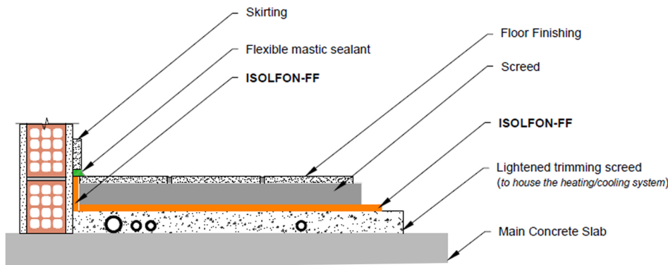
ISOLFON-FF : Εφαρμογή σε πλωτό δάπεδο από μπετόν.
