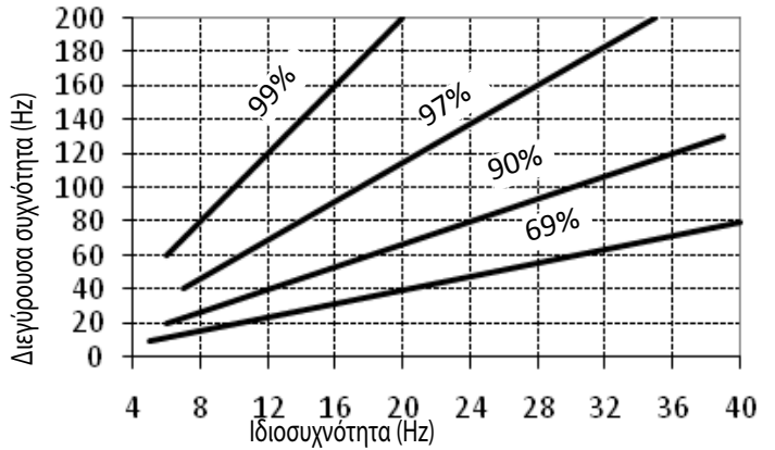
Διάγραμμα θεωρητικής μείωσης κραδασμών
