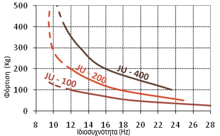
Διαγράμμά Φορτίου - Ιδιοσυχνότητας
