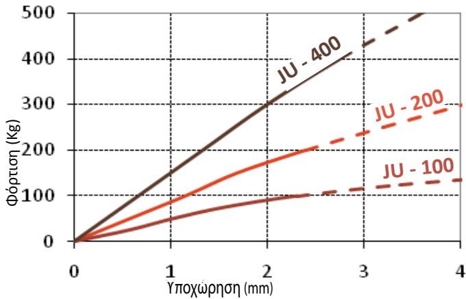
Διαγραμμα Φορτίου - Υποχώρησης
